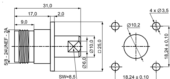
JC3.660.197 N-50KF-7 (диаметр=6)
