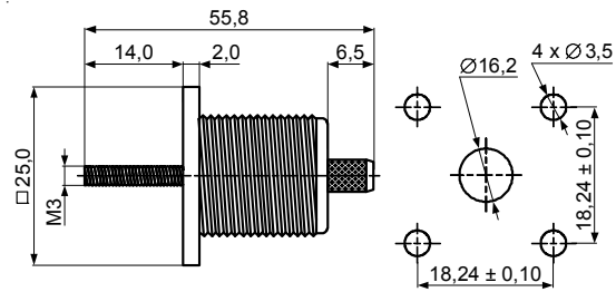
JC3.650.224 N-CF-3-C SYV-50-3 RG-58/U
