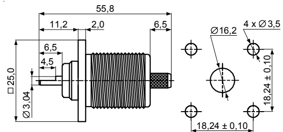
JC3.650.225 N-CF-3-D SYV-50-3 RG-58/U
