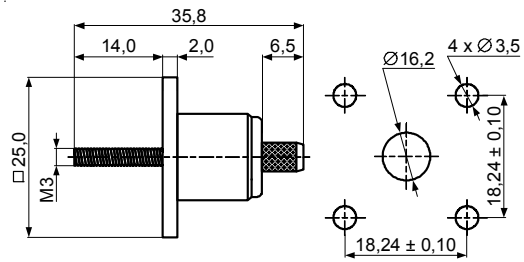
JC3.650.222 N-CF-3-A SYV-50-3 RG-58/U
