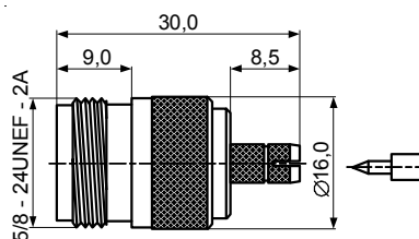
JC3.660.186-1 N-C-K3 SYV-50-3 RG-58/U
