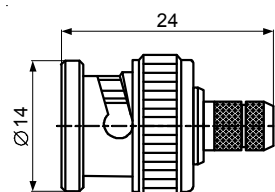
JC3.650.015/018 BNC-C-75J3/75J5/75J7 SYV-75-3 SYV-75-5-1 SYV-75-7
